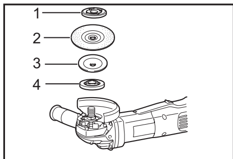
► 1. Contre-écrou 2. Meule flexible 3. Tampon d'ap-p 4. Bague interne
